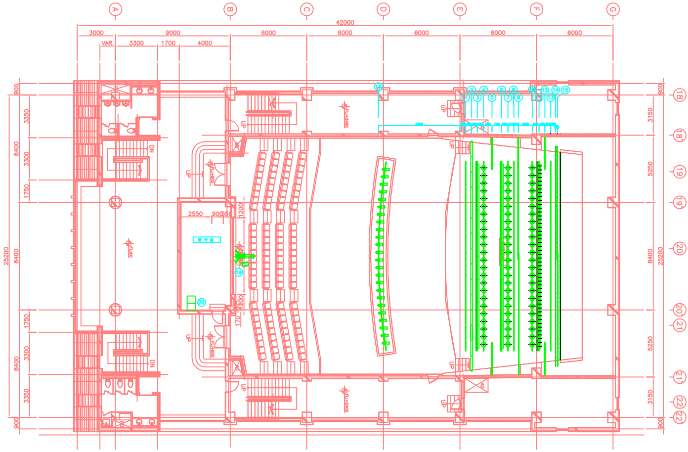
무대장치 천정평면 배치도 S : 1 / 100
